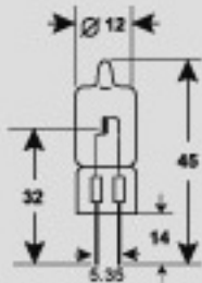
灯泡示意图(单位:毫米)
