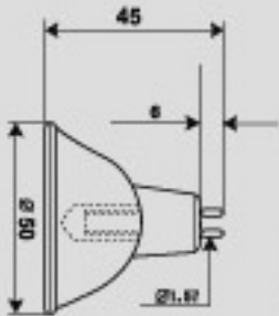
灯泡示意图(单位:毫米)
